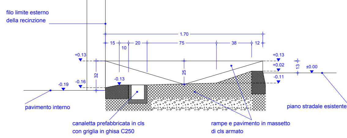
Sezione A-A
