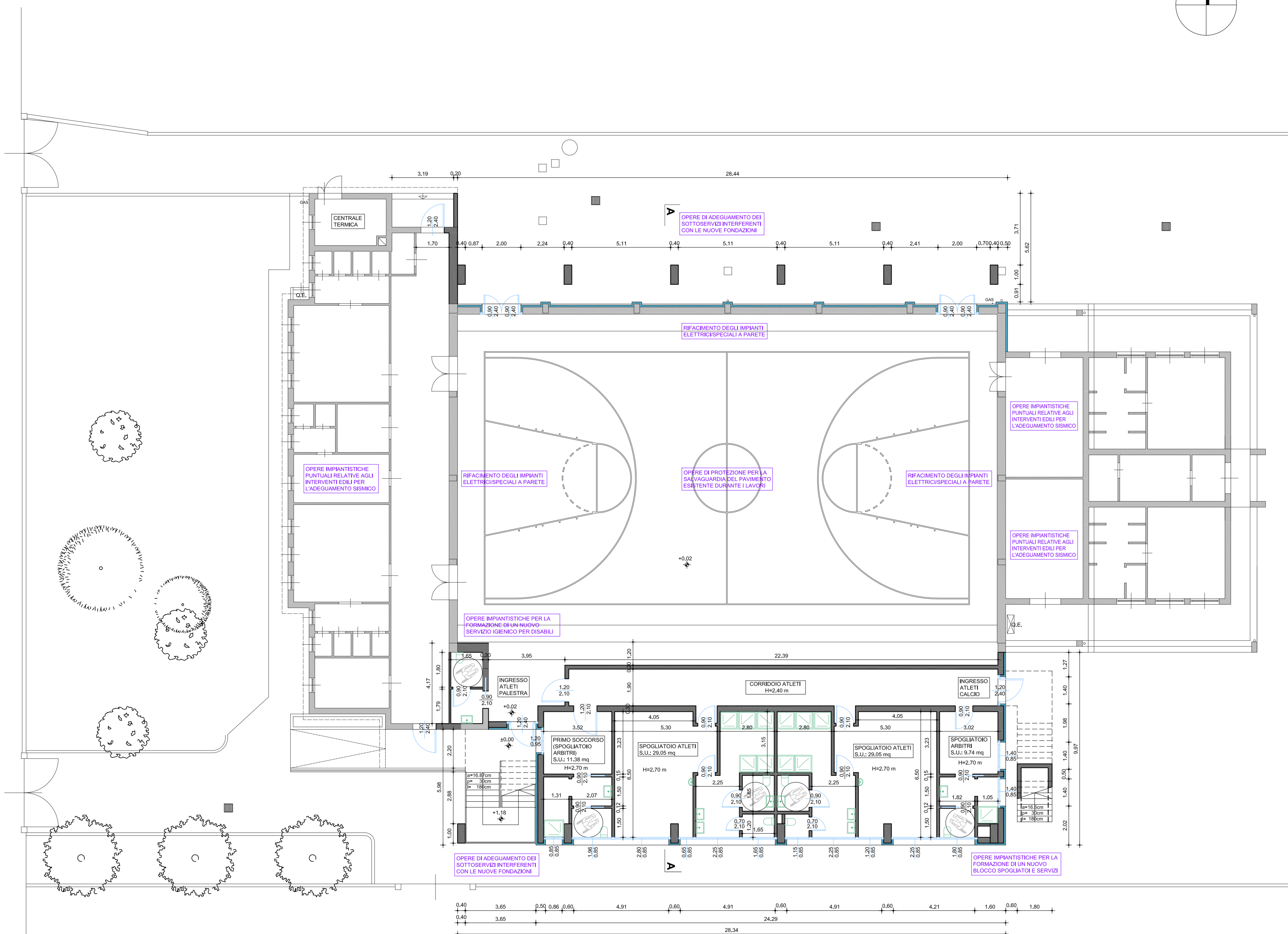
PIANTA PIANO TERRA
